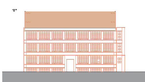
ANSICHT-OST M 1:200
