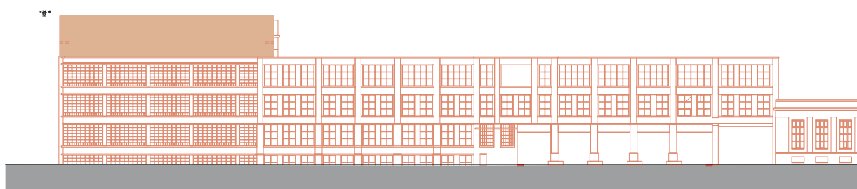
ANSICHT-NORD M 1:200
