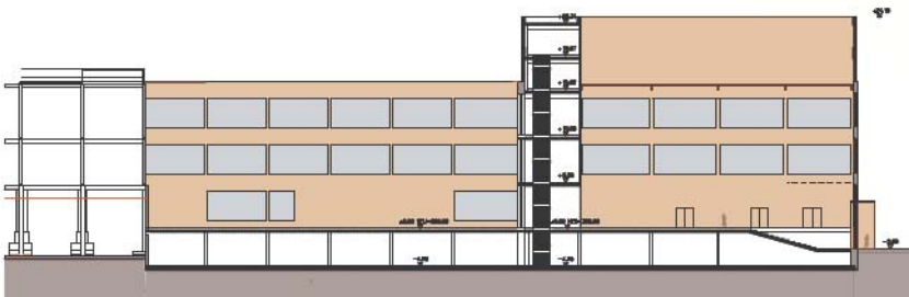
SCHNITT 3-3 M 1:200
