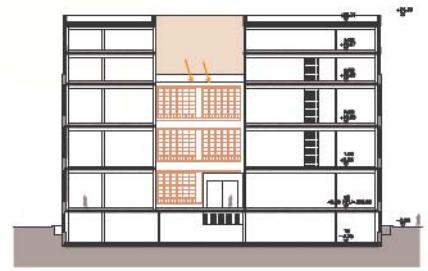
SCHNITT 1-1 M 1:200
